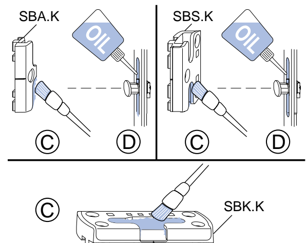
Bild 3: Schließbleche
