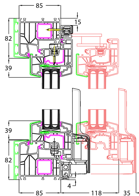
TWINSET 8000 SCHIEBEFLÜGEL
