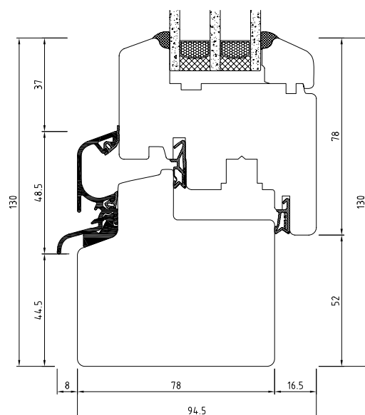
HOLZFENSTER IV 78 PROFILSCHNITT
