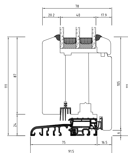
HOLZFENSTER IV 78 MIT HAUSTÜRSCHWELLE
