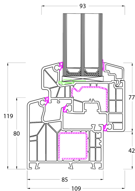
IDEAL DESIGN RAHMEN MIT FLÜGEL
