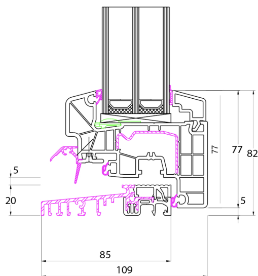
IDEAL DESIGN BALKONTÜRE MIT FLACHER SCHWELLE
