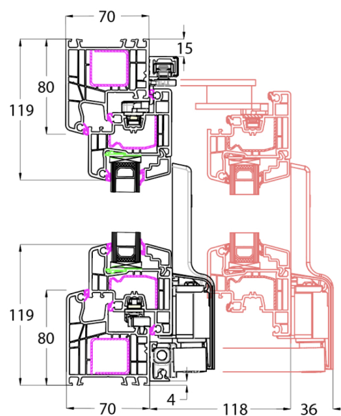
IDEAL 4000 HÖHENSCHNITT
