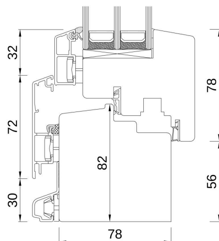
IDEALU Classicline IV 78 RAHMEN MIT FLÜGEL
