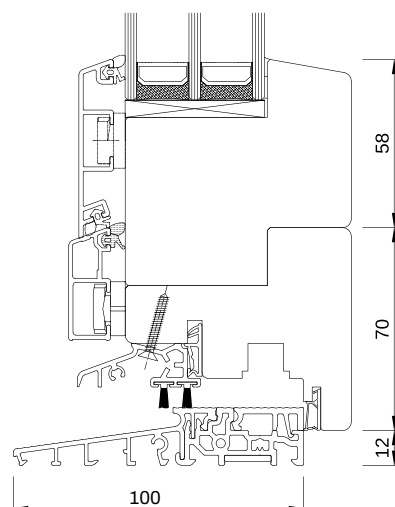
IDEALU Classicline IV 78 BALKONTÜRE MIT FLACHER SCHWELLE
