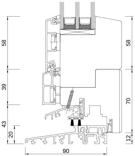
IDEALU Classicline IV 68 BALKONTÜRE MIT FLACHER SCHWELLE
