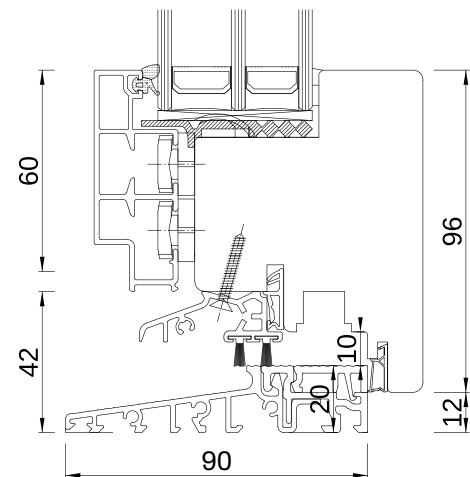
IDEAL PLANO BALKONTÜRE MIT FLACHER SCHWELLE
