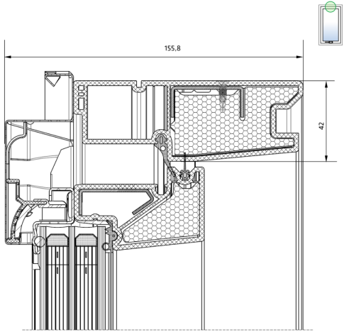
ANSICHT OBEN: SCHWINGFLÜGEL 3-FACH VERGLASUNG
