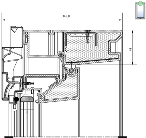
ANSICHT OBEN: SCHWINGFLÜGEL 2-FACH VERGLASUNG
